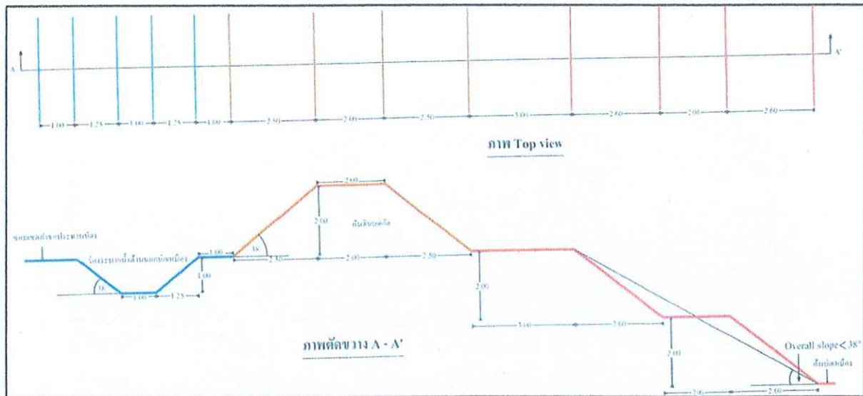
รูปที่ 1 ภาพแสดงการออกแบบเหมือง
