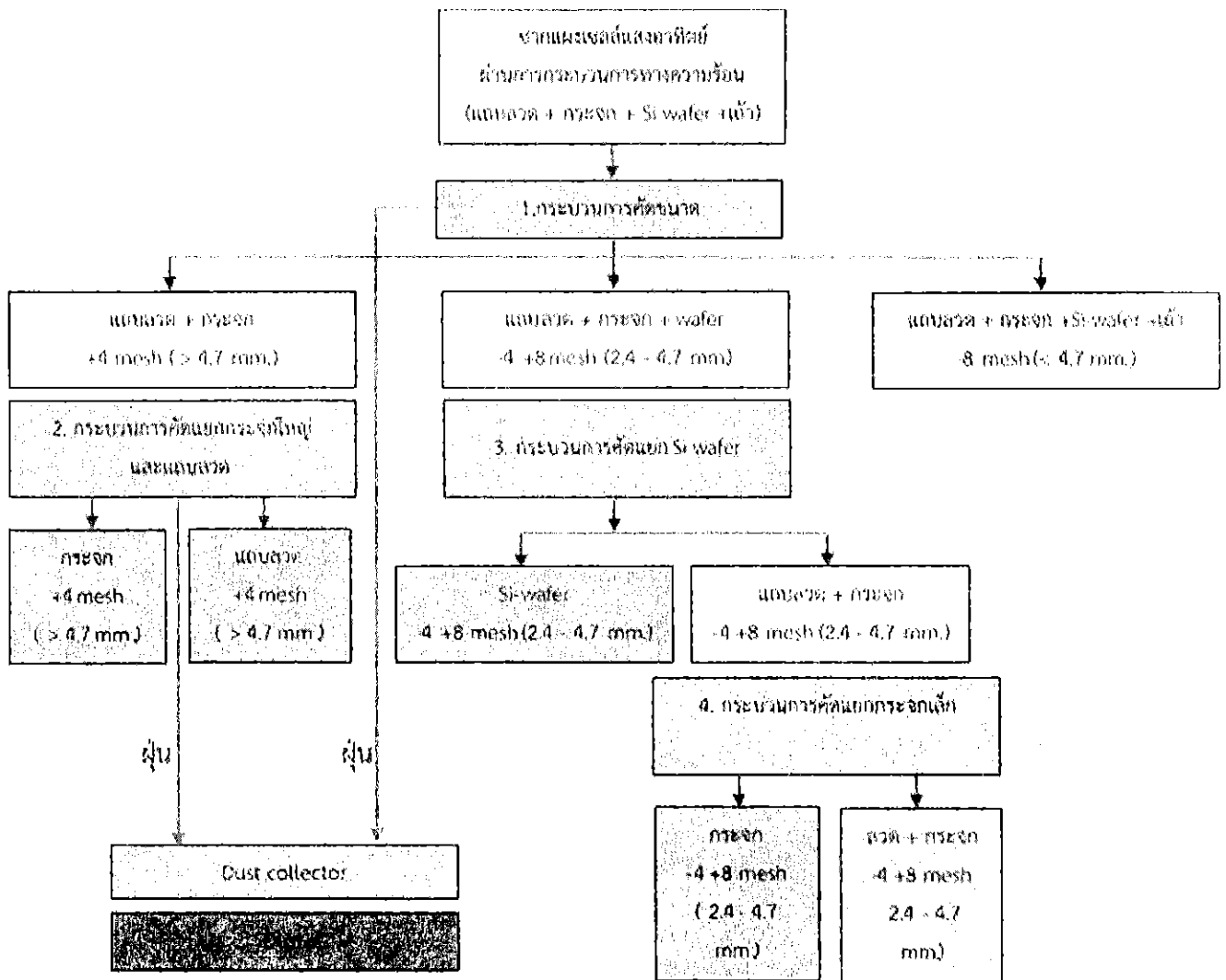
รูปที่ 1 ขั้นตอนโดยสังเขปของเครื่องจักรและอุปกรณ์แต่งแร่สำหรับการคัดแยก ซากแผงเซลล์แสงอาทิตย์ที่ผ่านกระบวนการทางความร้อนมาแล้ว
