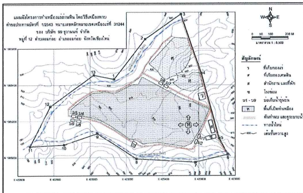
รูปที่ ๒ แผนผังโครงการทำเหมืองแร่ถ่านหิน โดยวิธีเหมืองทาบ คำขอประทานบัตรที่ ๑/๒๕๔๓
